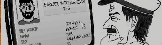
Näotuvastus
